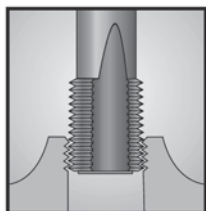
Vyřezat pomocný závit
