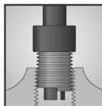
Našroubovat závitovou vložku
